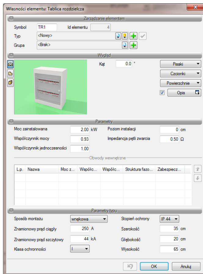
Rys. 13. Okno Własności elementu: Tablica rozdzielcza
